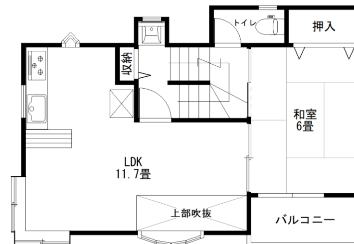
2階
